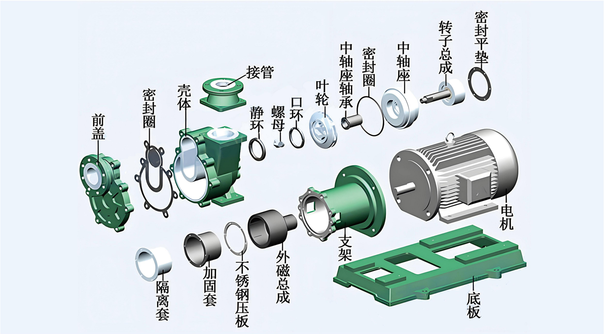
产品结构解析图
